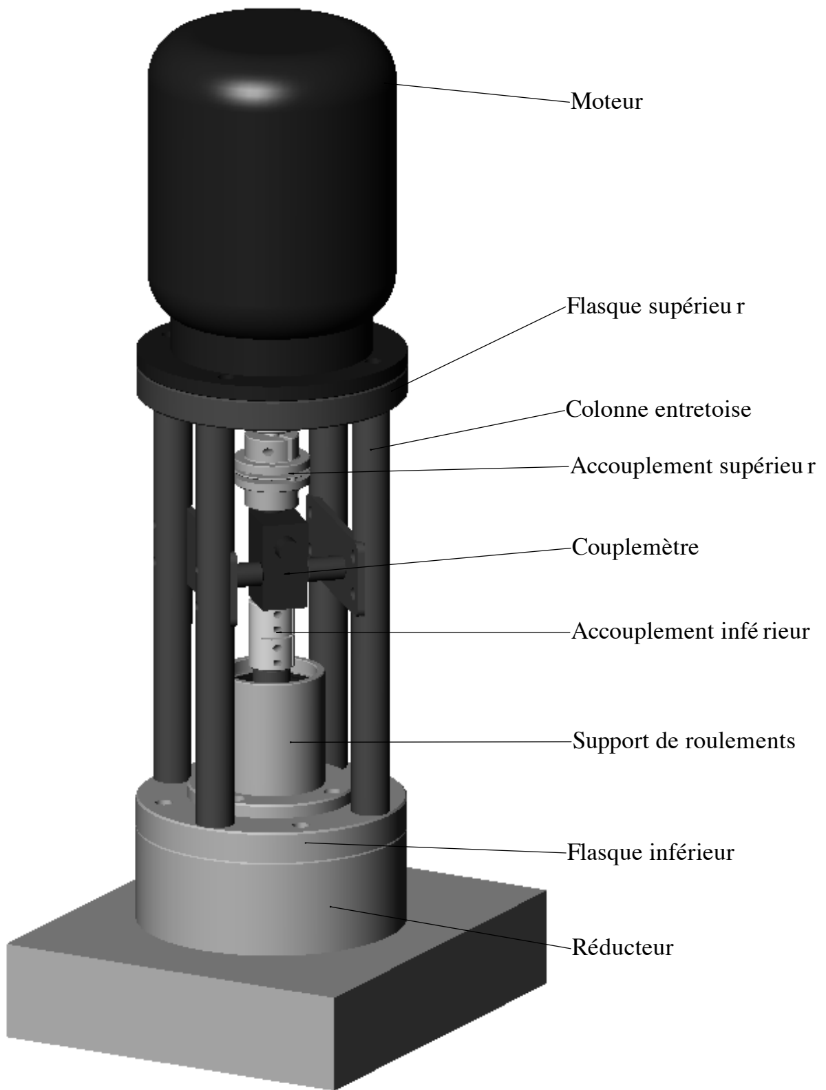
Vue d'ensemble du montage du couplemètre
